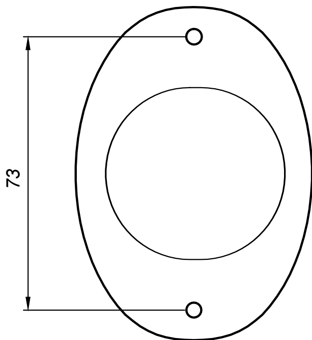
Пластиковая вставка
